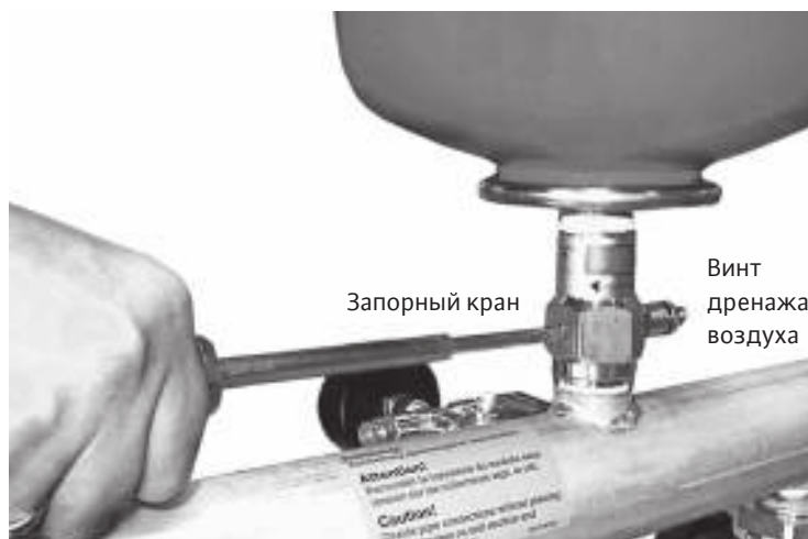
Рис. 2б Обслуживание мембранного бака и проверка давления его наддува
